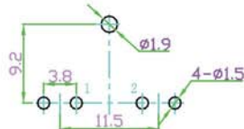
印制板开孔尺寸(±0.1mm)
